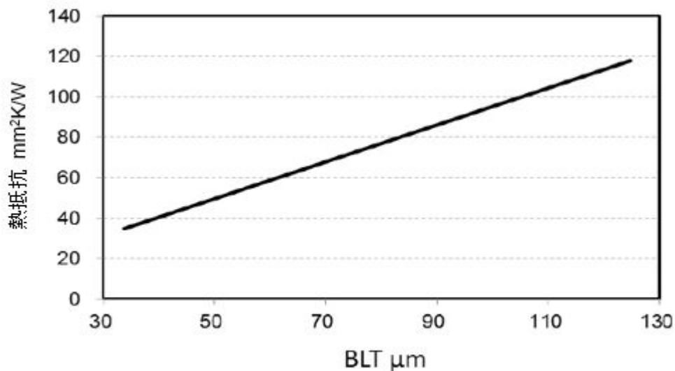
図 TIG1500の厚み (um)と熱抵抗の関係 (mm 2 K/W)
